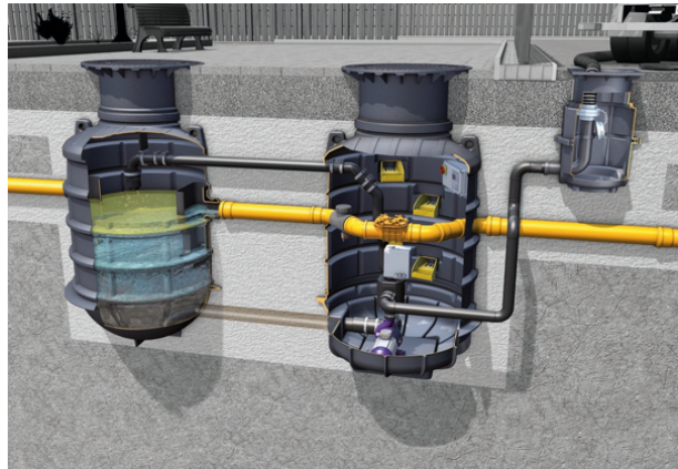
Einbaubeispiel Fettabscheider EasyClean ground Auto Mix & Pump
